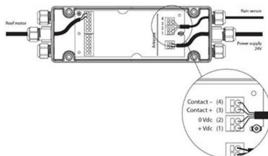
io Motorsteuerung
