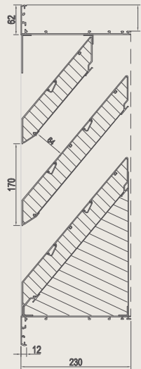
Dessin de coupe
