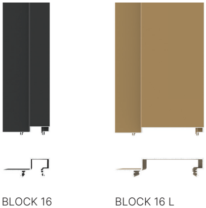
De gevelvlakken met lamellen zijn een afwisseling van BLOCK 16 en BLOCK 16L-profielen
