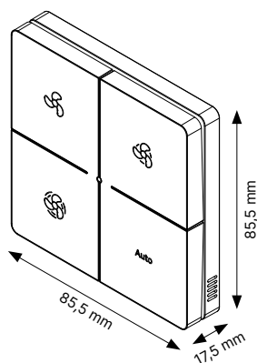
38444 - Interrupteur à quatre positions
