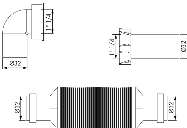
Kit de siphon (code d'article : 17792)
