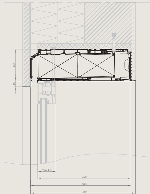
Vb. Endura Twist horizontaal inblaas naar onder met pleisterprofiel
