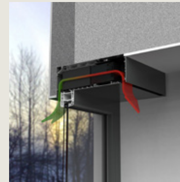
Inblaas naar onder
