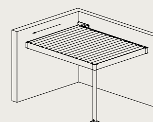
volledige muur (gevelmontage) span en pivot
