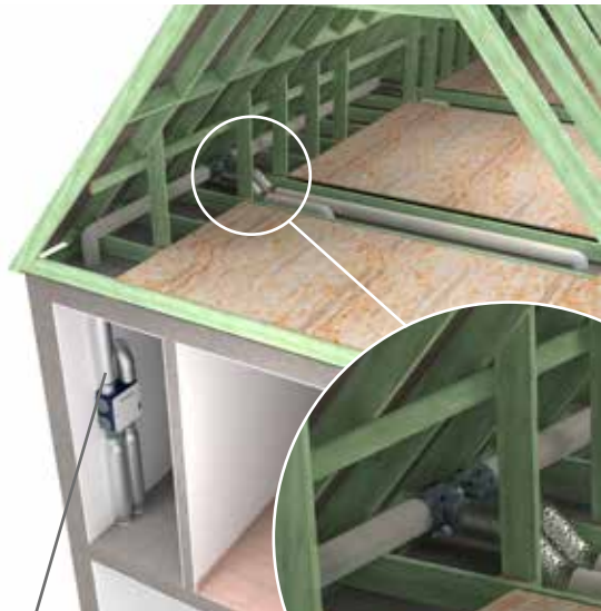
Kolektor zaworowy nie musi być zamontowany na wentylatorze; może być też zainstalowany z dala od niego. Pozwala to na osiągnięcie tego samego rezultatu przy mniejszej liczbie kanałów wentylacyjnych.
