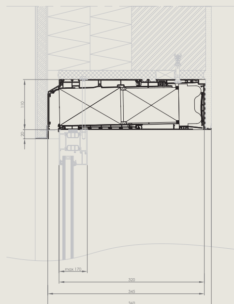
Ex. Endura Twist horizontal pulsion vers le bas avec profil de plâtre
