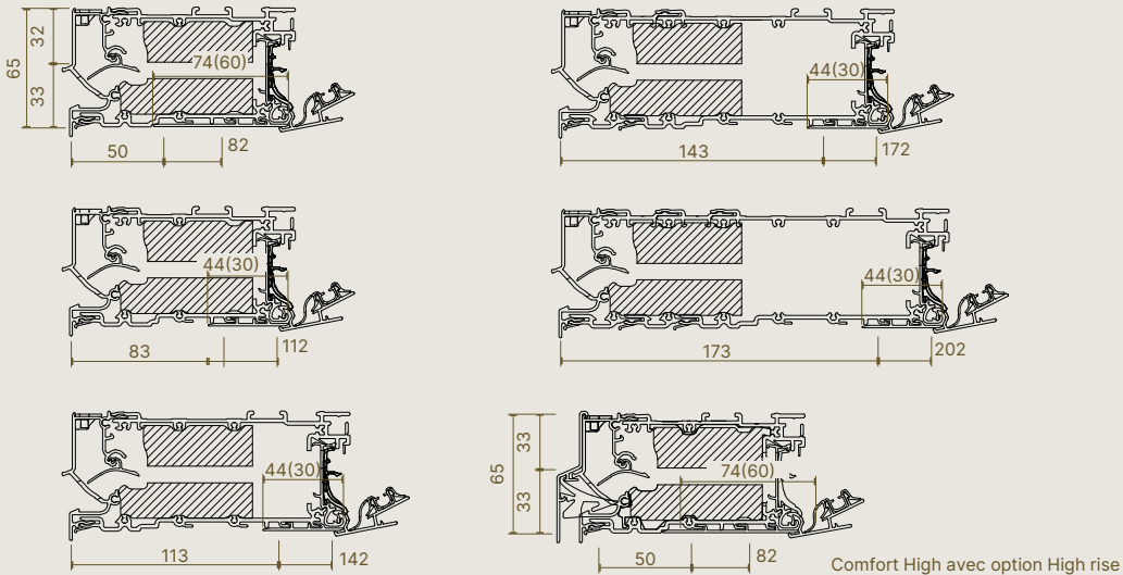
Dessins de coupe l'Invisivent® COMFORT High
