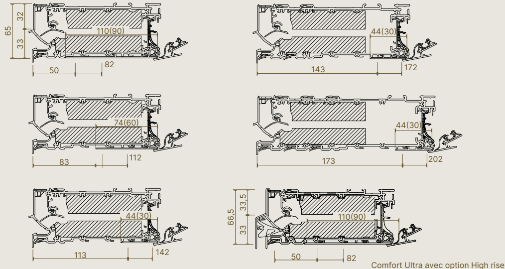
Dessins de coupe l'Invisivent® COMFORT Ultra
