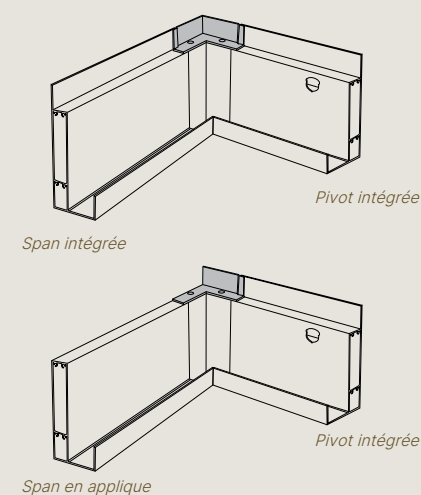
Capuchon d'angle supérieur avec profil de raccordement au mur
