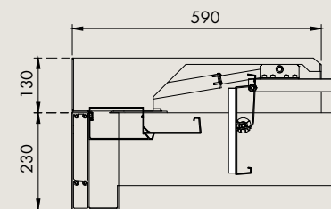
Configuration sans profile de raccordement au mur
