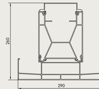
Pivot gekoppeld
