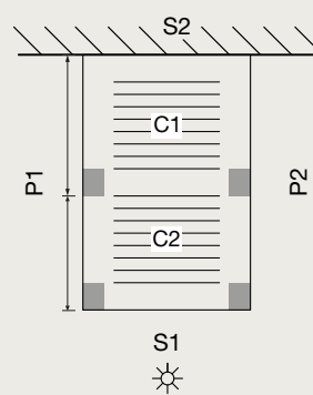
Gevelmontage span
