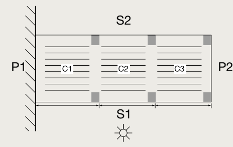
Gevelmontage pivot
