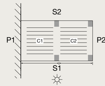
Gevelmontage pivot
