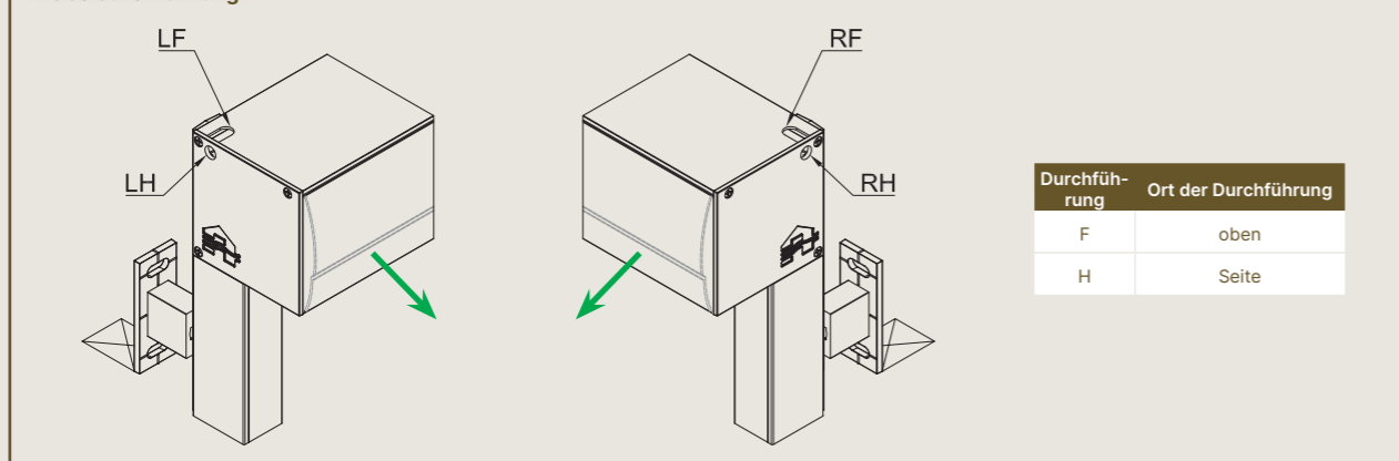
Kabeldurchführung
