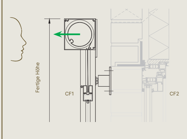
Fixscreen® 100 – Vorbauzeichnung vom Mauerwerk
