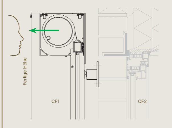
Fixscreen® 150 – Vorbauzeichnung vom Mauerwerk
