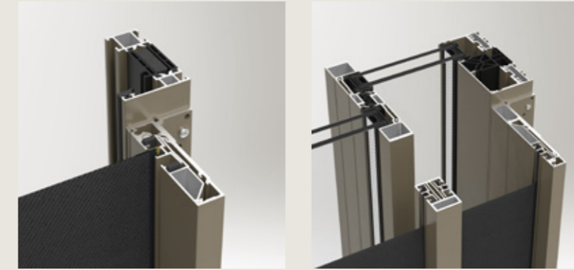
S.WF in Kombination mit einem Fenster
