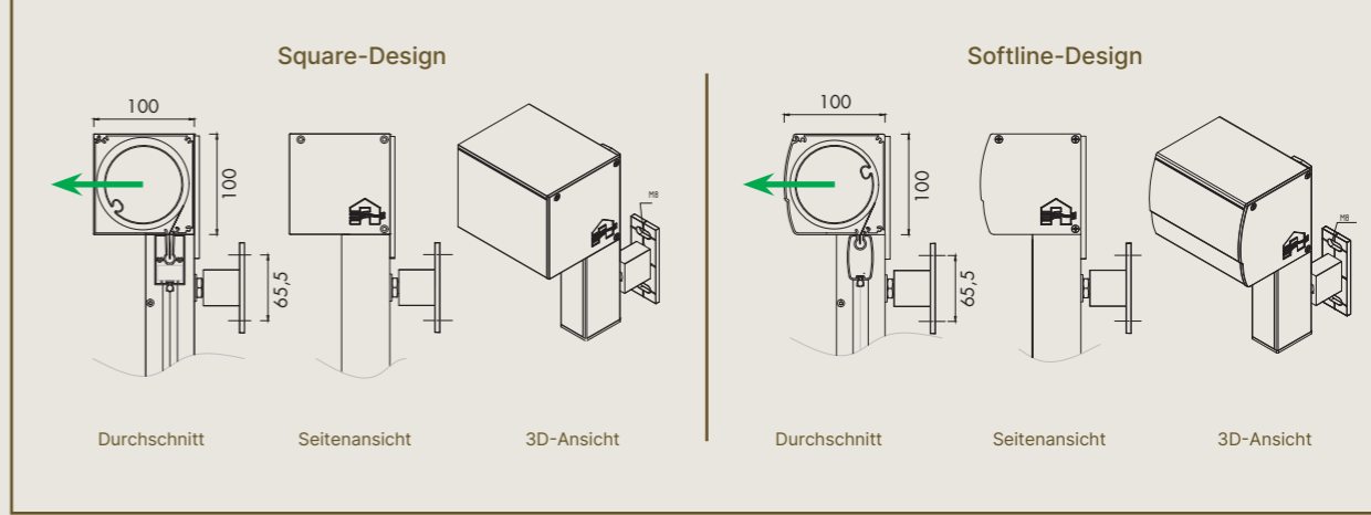
Fixscreen® 150 – Kassette
