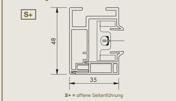
Seitenführung
