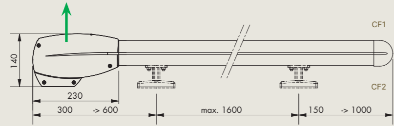
Seitenansicht
