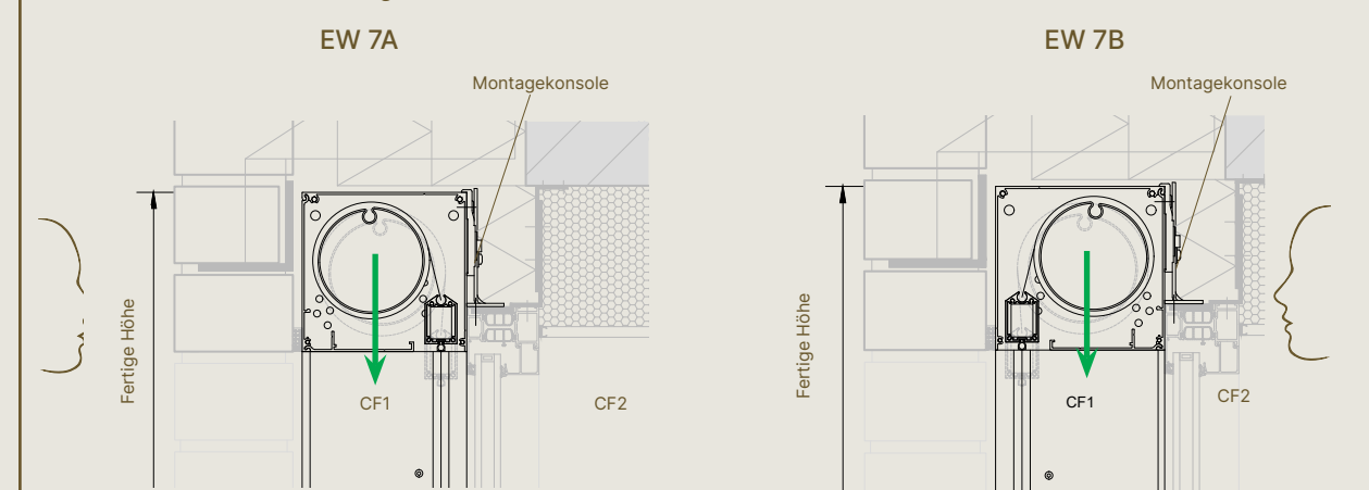
Fixscreen® 150 – Einbauzeichnung Putz
