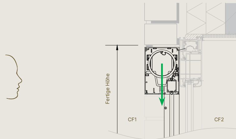
Vorbauzeichnung vom Mauerwerk
