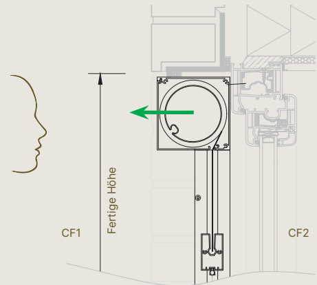
Fixscreen® 100 – Vorbauzeichnung vom Mauerwerk
