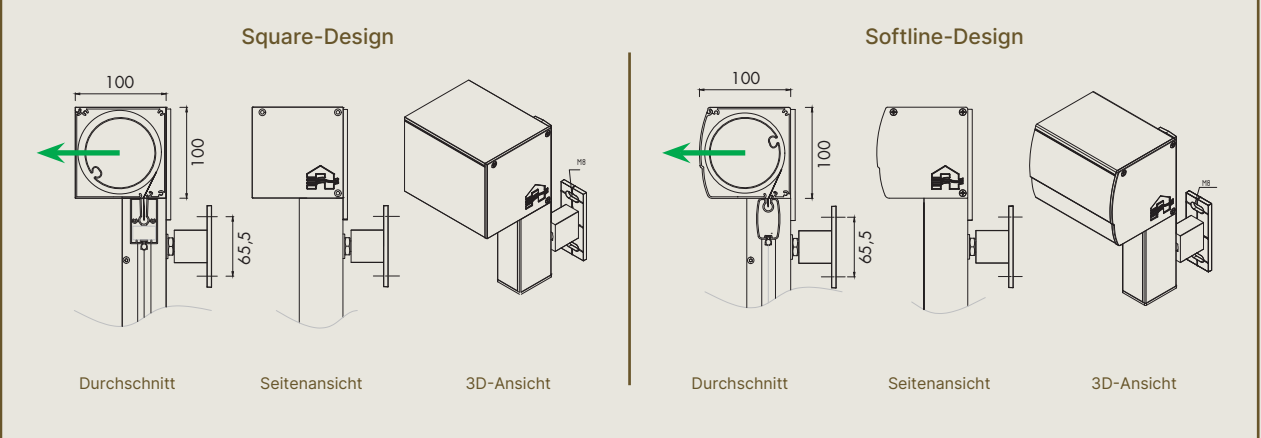
Fixscreen® 150 – Kassette
