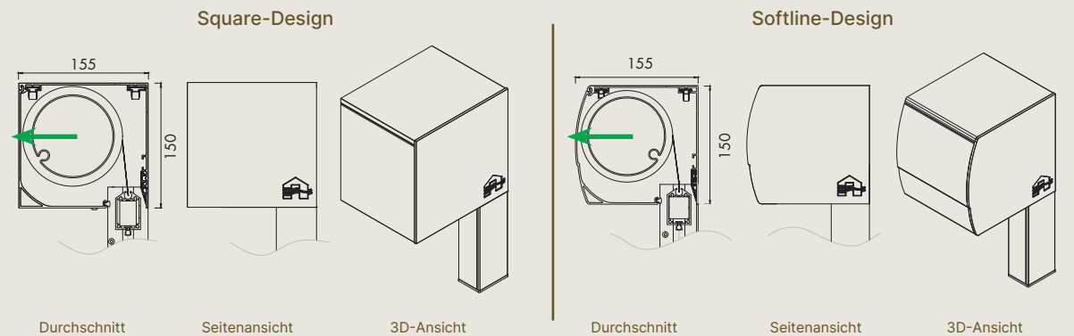
Fixscreen® 150 – Kassette
