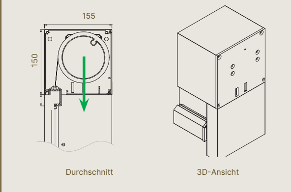
Fixscreen® 150 – EW 7B F – Kassette
