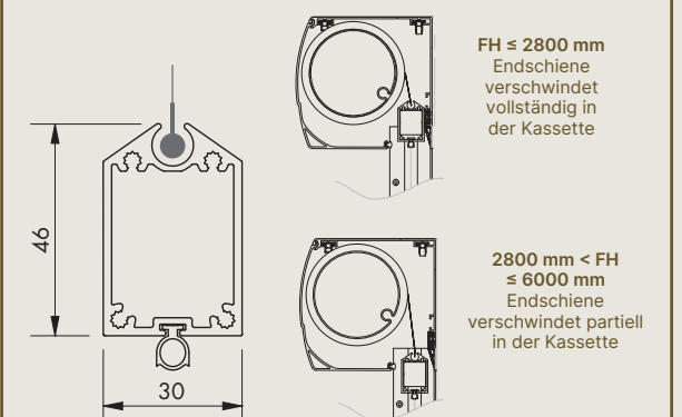
Fixscreen® 150 – Endschiene
