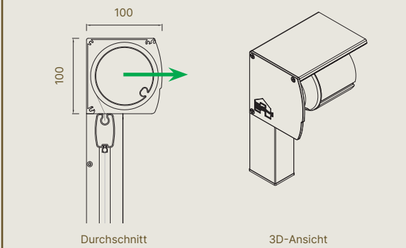
Fixscreen® 100 – Kassette
