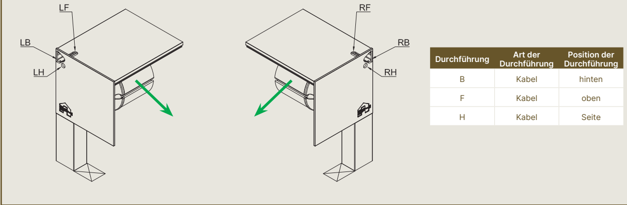
Fixscreen® 150 – Kabeldurchführung
