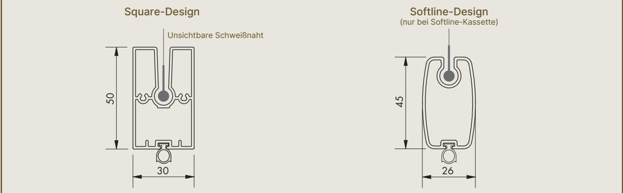
Fixscreen® 150 – Endschiene
