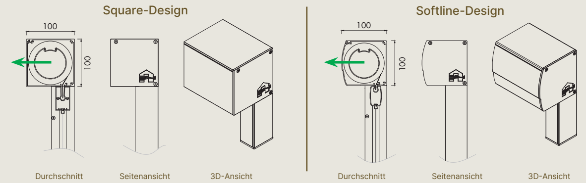
Fixscreen® 150 – Kassette
