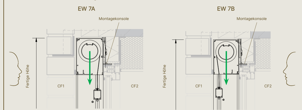
Fixscreen® 100 Slim – Einbauzeichnung Putz
