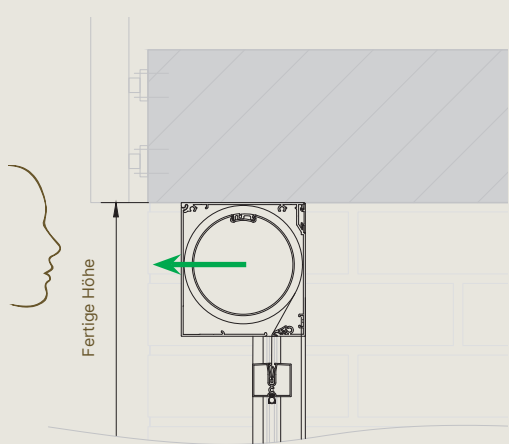
Large – Vorbauzeichnung vom Balkon
