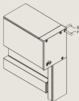
Kabeldurchführung B/H
