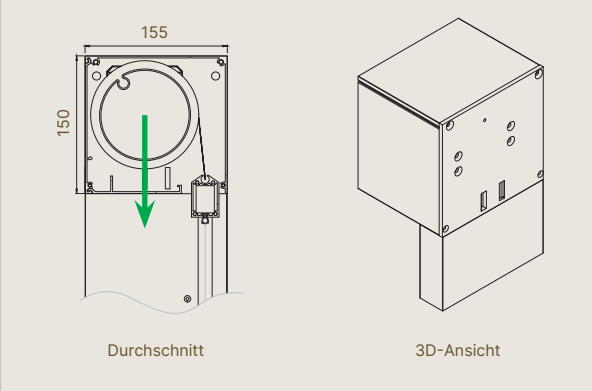
Kabeldurchführung – EW 7A F
