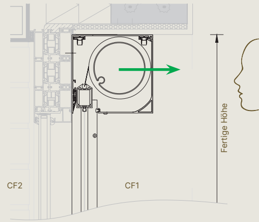
Fixscreen® 150 – Vorbauzeichnung der Innenanwendung
