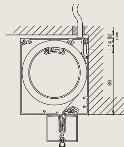
Hakenprofil
