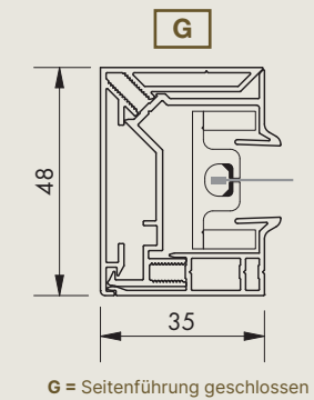
Seitenführungen
