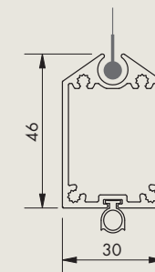
Endschiene
