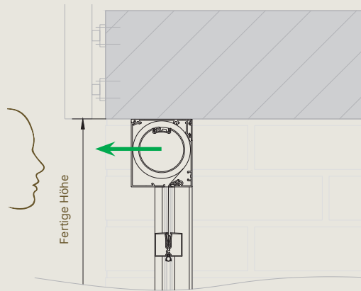
Small – Vorbauzeichnung vom Balkon
