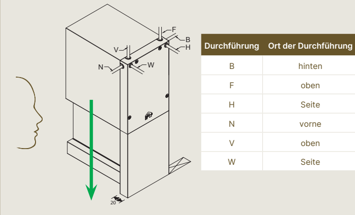
Kabeldurchführung
