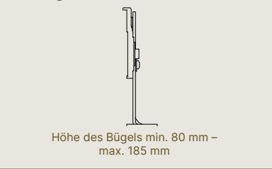
Montagekonsole
