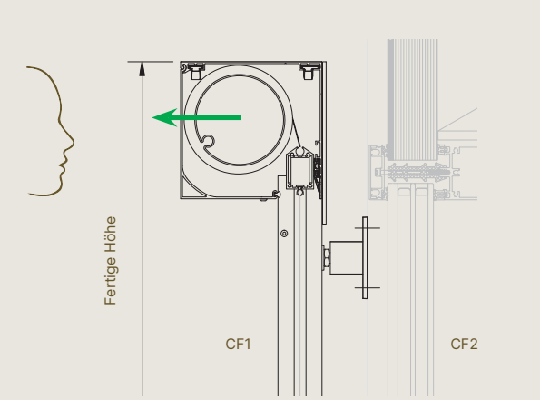
Fixscreen® 150 – Vorbauzeichnung Vorhangfassade
