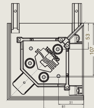
Eckbügel (Position der Bohrlöcher)
