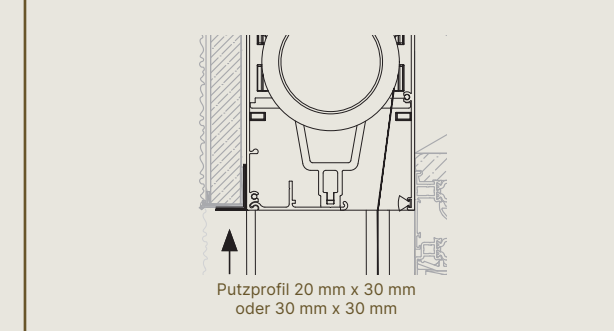
Putzprofil
