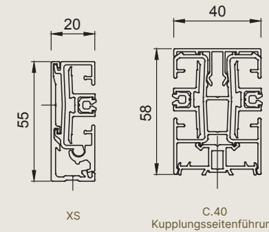
Seitenführungen
