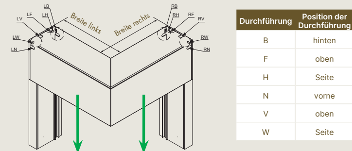
Kabeldurchführung
