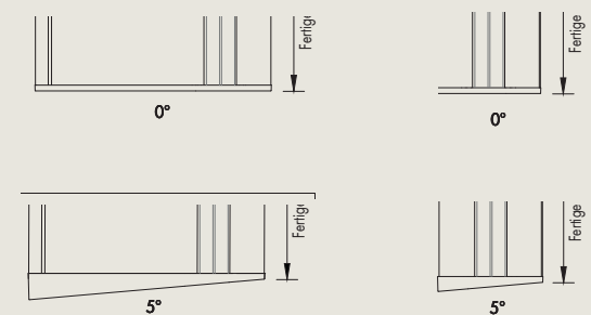
Grundplatte Seitenführung
