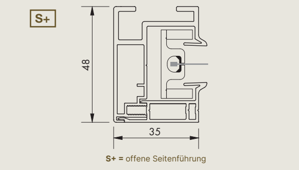
Seitenführung
