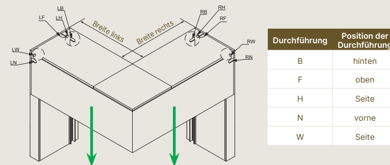
Kabeldurchführung
