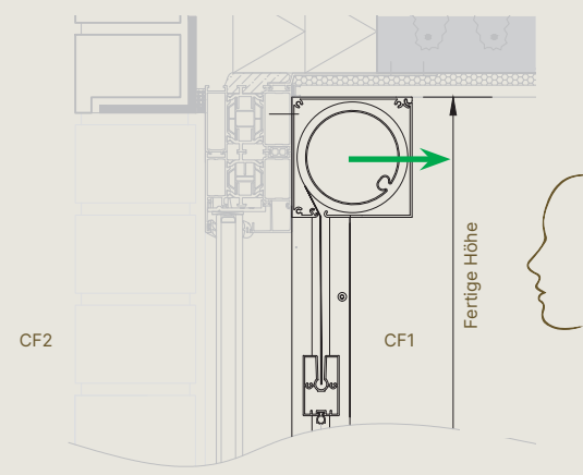
Fixscreen® 100 – Vorbauzeichnung der Innenanwendung
