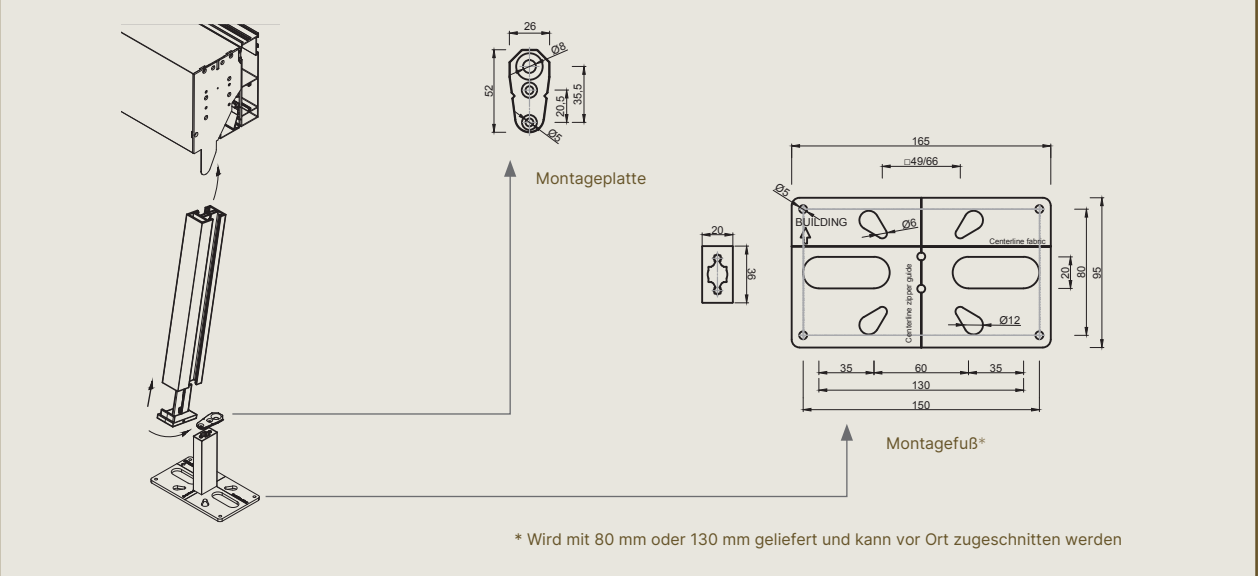
Befestigungsmöglichkeiten
