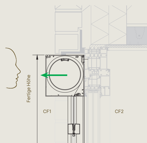
Large – Vorbauzeichnung vom Mauerwerk
