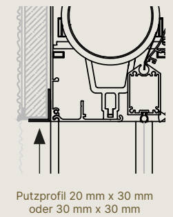
Putzprofil
