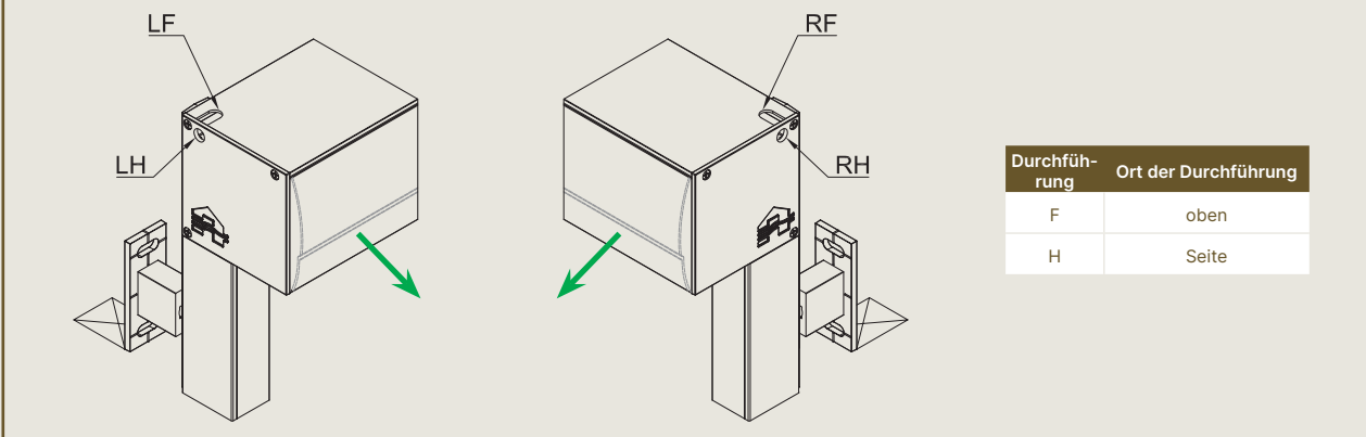
Grundplatte Seitenführung
