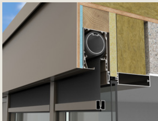
Einbau-Anwendung
