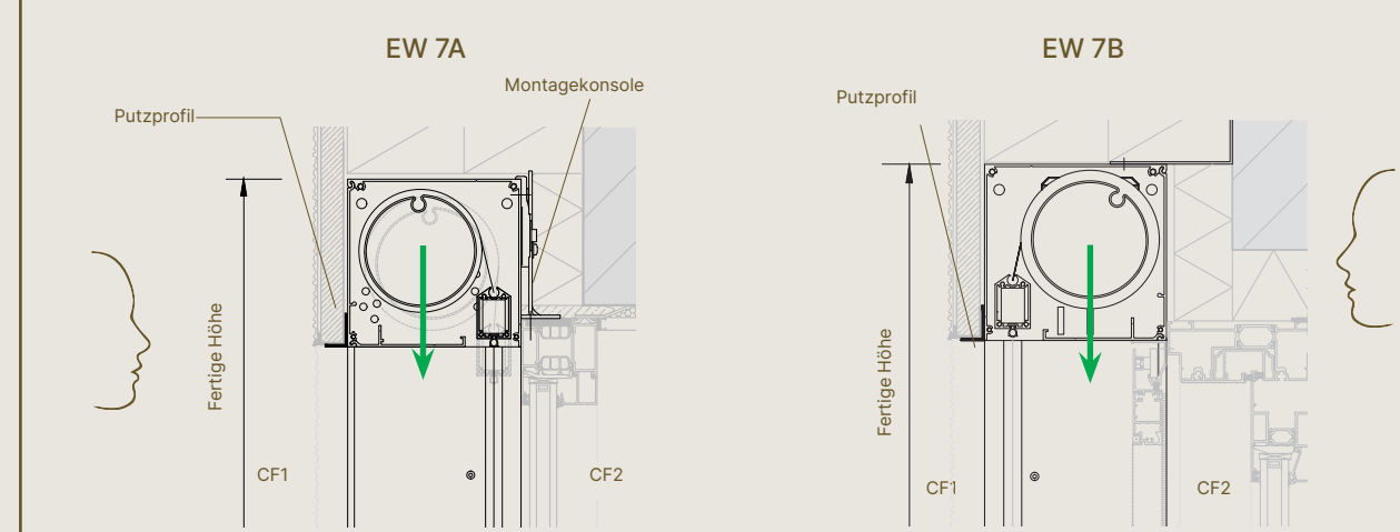
Fixscreen® 150 – Einbauzeichnung Putz
