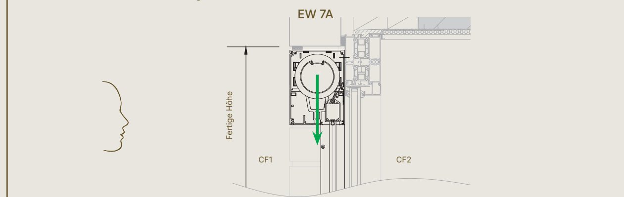
Fixscreen® 100 Slim – Vorbauzeichnung vom Mauerwerk
