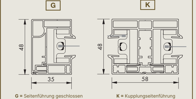
Seitenführungen
