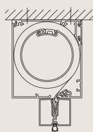
Füllprofil
