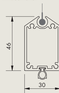
Endschiene
