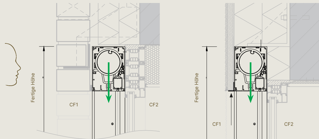
Vorbauzeichnung vom Mauerwerk
