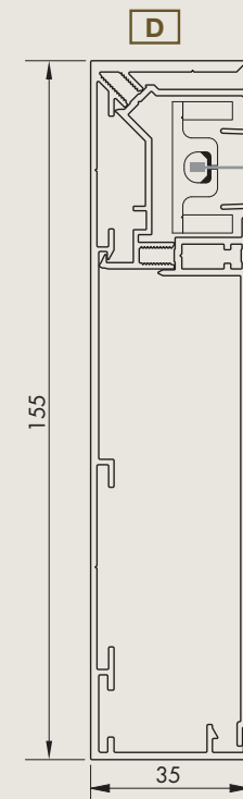
D = tiefe Seitenführung (Standard)
