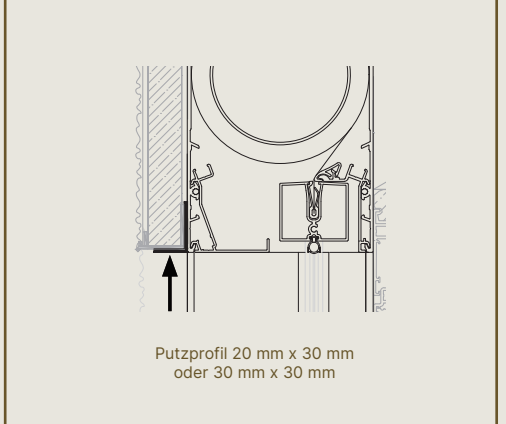
Putzprofil
