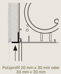
Putzprofil
