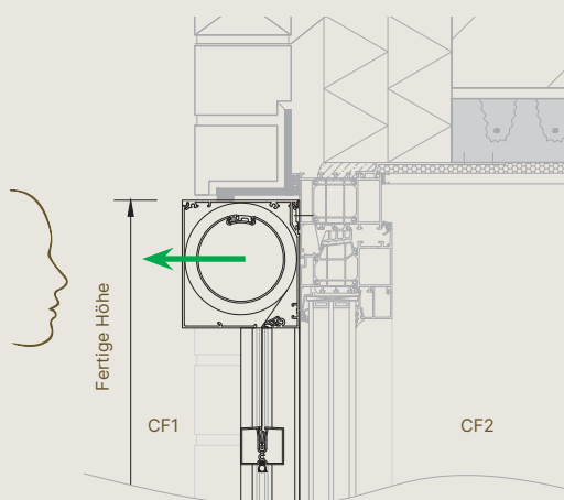
Medium – Vorbauzeichnung vom Mauerwerk
