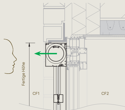
Small – Vorbauzeichnung vom Mauerwerk
