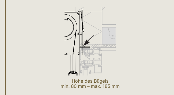
Montagekonsole
