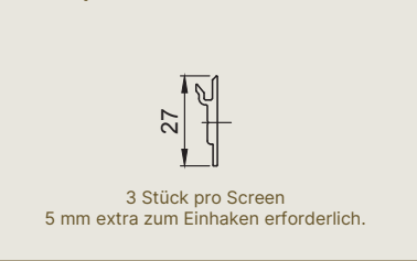
Hakenprofil
