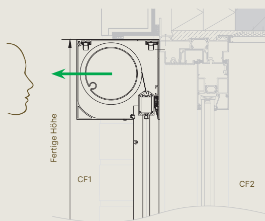
Fixscreen® 150 – Vorbauzeichnung vom Mauerwerk
