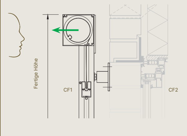
Fixscreen® 100 – Vorbauzeichnung Vorhangfassade
