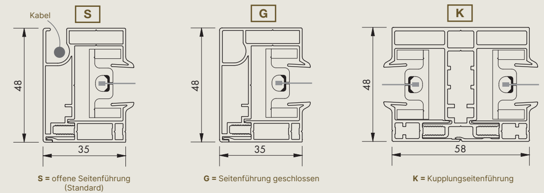
Seitenführungen
