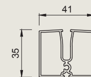
Grundplatte Seitenführung
