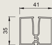
Endschiene
