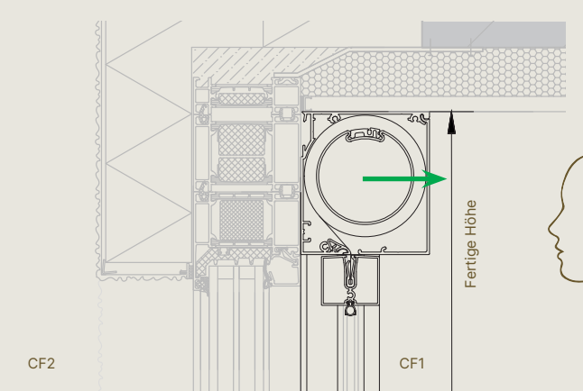
Small – Vorbauzeichnung der Innenanwendung
