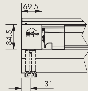
Vorderansicht
