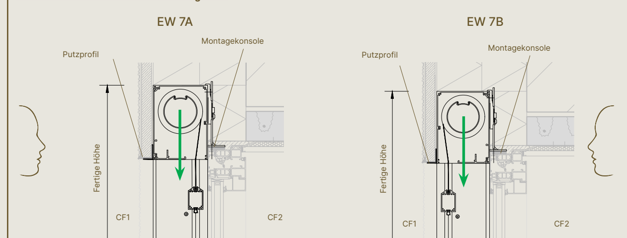
Fixscreen® 100 Slim – Vorbauzeichnung vom Mauerwerk
