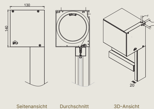
Seitenansicht Durchschnitt 3D-Ansicht
