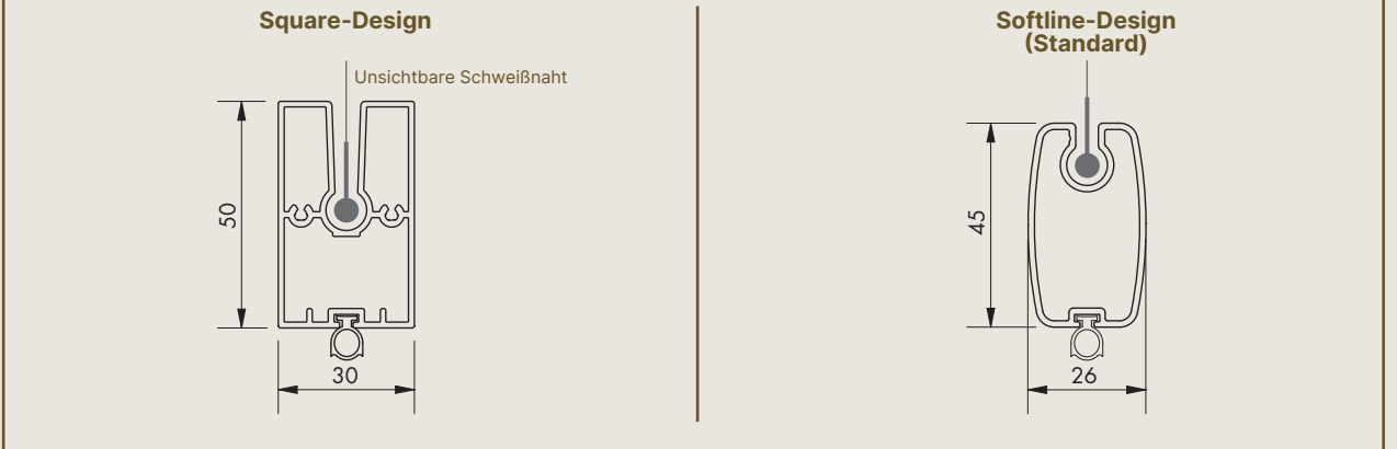
Fixscreen® 150 – Endschiene
