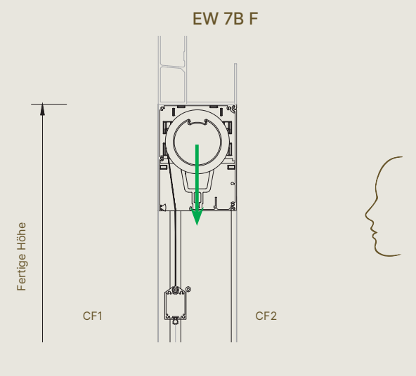
Einbauzeichnung Algarve
