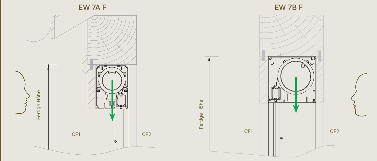
Einbauzeichnung Balkon
