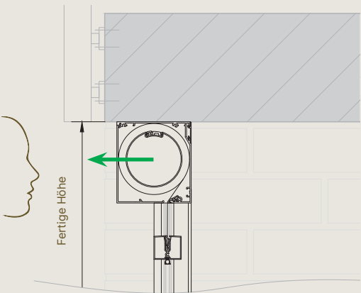
Medium – Vorbauzeichnung vom Balkon
