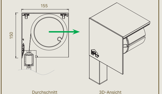
Fixscreen® 150 – Kassette
