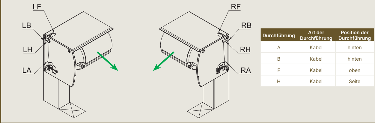
Fixscreen® 100 – Kabeldurchführung
