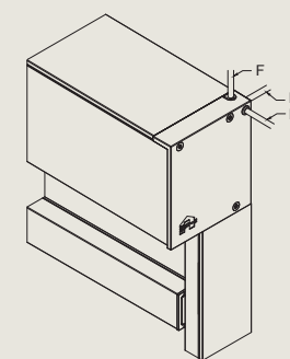
Kabeldurchführung B/F/H
