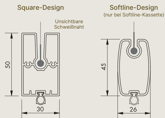
Fixscreen® 100 – Endschiene
