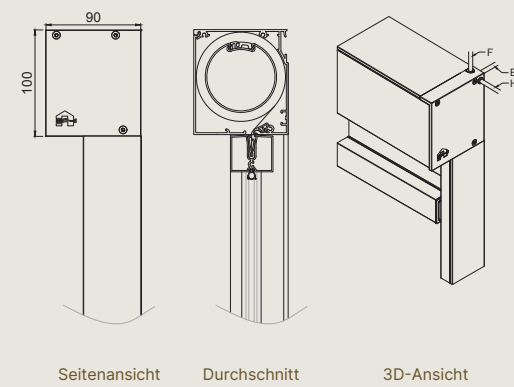
Seitenansicht Durchschnitt 3D-Ansicht
