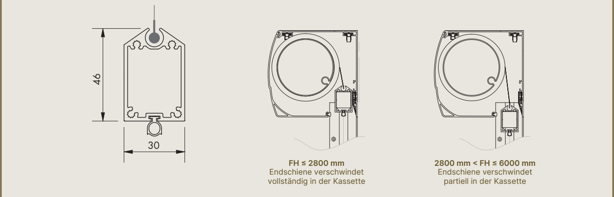
Fixscreen® 150 – Endschiene
