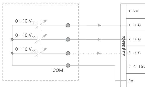
Commande externe
