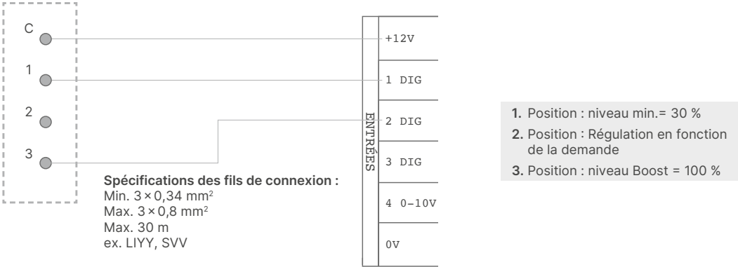
Interrupteur externe
