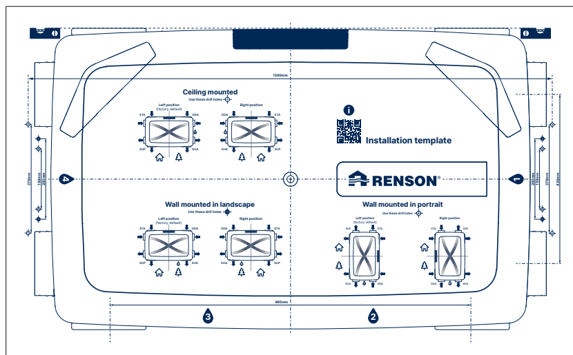
Montage au plafond avec QuickFix – Position dans la pièce (unité en mm) – Configuration des trous de l'équerre QuickFix.
