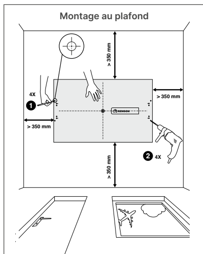
Montage au plafond avec QuickFix – Position dans la pièce (unité en mm) – Configuration des trous de l'équerre QuickFix.
