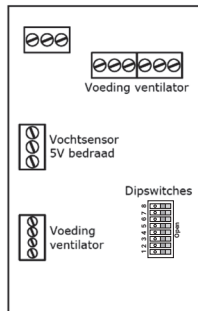
Printplaat
