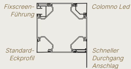
Pfosten
