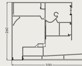
Pivot freistehend
