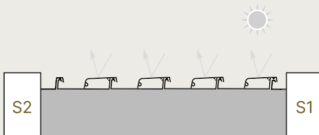
Geschlossenes Dach
