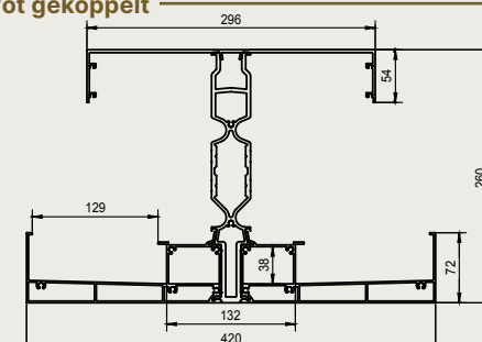
Pivot gekoppelt
