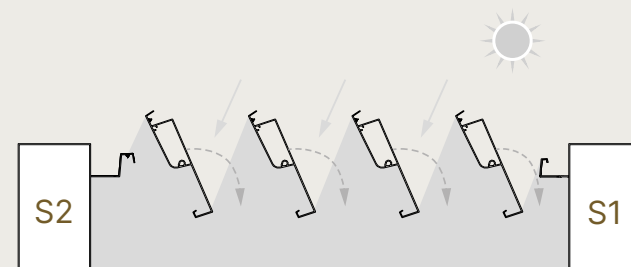
Indirekte Sonneneinstrahlung
