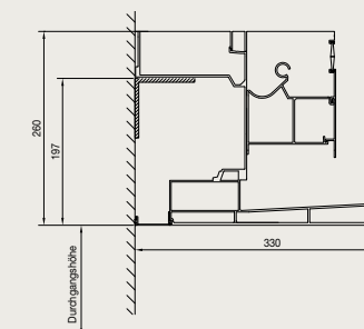
Pivot Fassadenmontage
