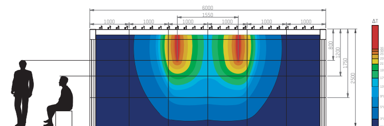
2 lames Lineo heat avec 1 élément de chauffage
