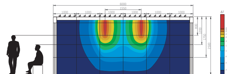
2 lamelle Lineo Heat con 1 riscaldatore
