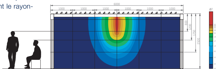
1 lame Lineo heat avec 1 élément de chauffage
