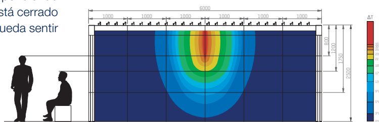
1 lama Lineo Heat con 1 calefacción
