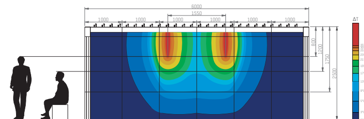
2 Lineo heat lamellen met 1 verwarming
