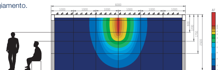
1 lamella Lineo Heat con 1 riscaldatore
