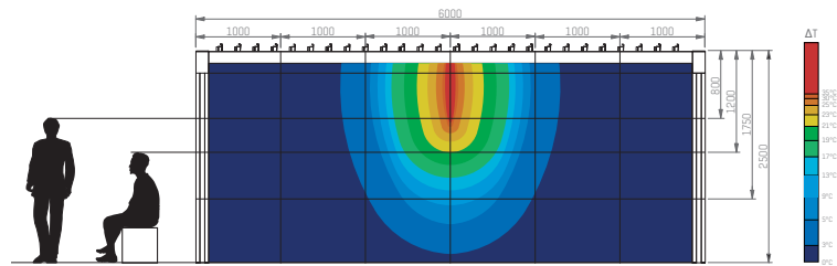
1 Lineo-heat Lamelle mit 1 Heizung
