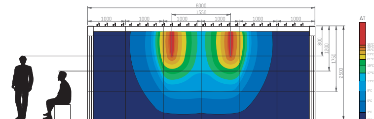
2 Lineo-heat Lamellen mit 1 Heizung
