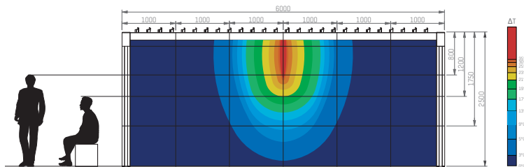
1 Lineo heat lamel met 1 verwarming
