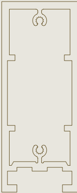
Ref. SD.100 Große freie Spannweite
