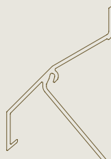
L.050CL Abschlusslamellen
