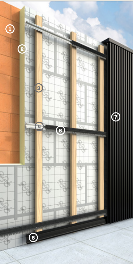
Sur un chevonnage bois ou une structure existante
