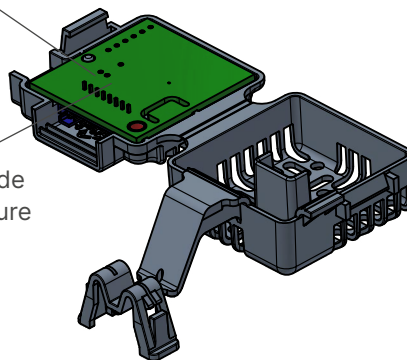
Capteur HR (capteur d'humidité)
