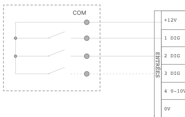
Interrupteur externe
