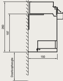
Span montage contre le façade
