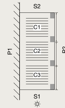
Montage contre la façade pivot
