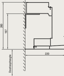
Pivot montage contre le façade
