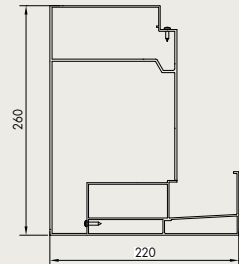
Pivot montage contre le façade
