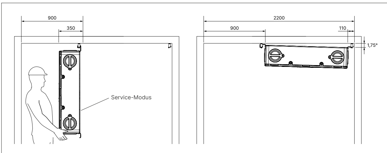
Deckenmontage mit QuickFix – Min. 900 mm erforderlicher Freiraum für optimalen Zugang bei der Wartung (Einheit in mm).
