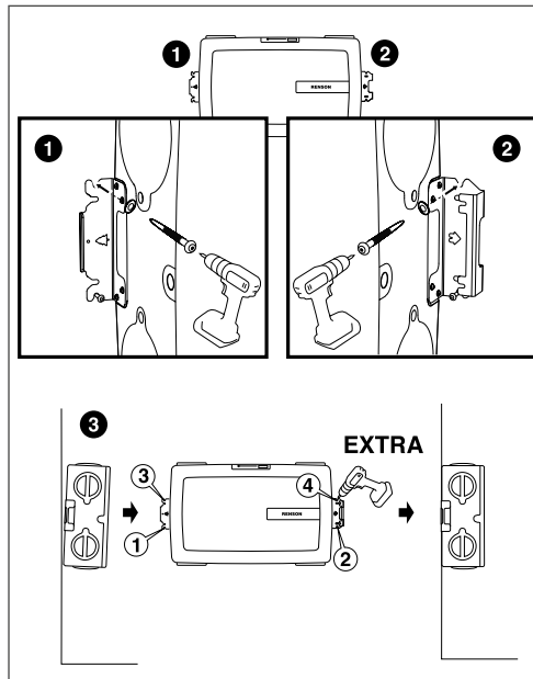
Horizontale Wandmontage – Schrauben festziehen.
