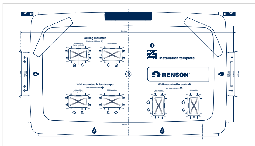
Horizontale Wandmontage (mit Schrauben und Dübeln) – Anordnung der Löcher auf der Bohrschablone.
