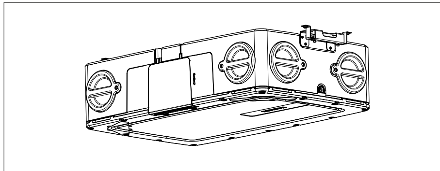
Deckenmontage mit QuickFix – Gerät am QuickFix befestigt.
