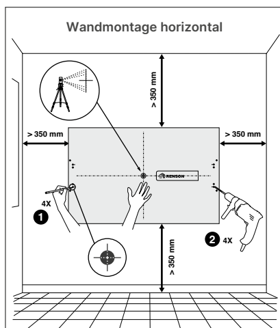
Horizontale Wandmontage (mit Schrauben und Dübeln) – Anordnung der Löcher auf der Bohrschablone.
