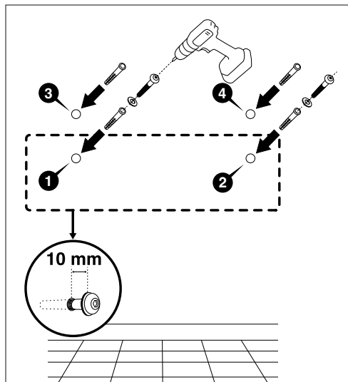
Horizontale Wandmontage – min. 1 cm Abstand zwischen Wand und Kopfbolzen zum Einhängen des Geräts.
