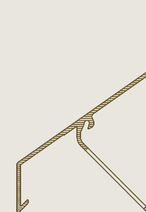
Ref. L.066 IM1 Lamel met geïntegreerde insectenwering
