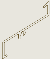
L.050HF Lamel met grote doorlaat
