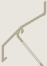
L.050IM2 Lamel met geïntegreerde insectenwering
