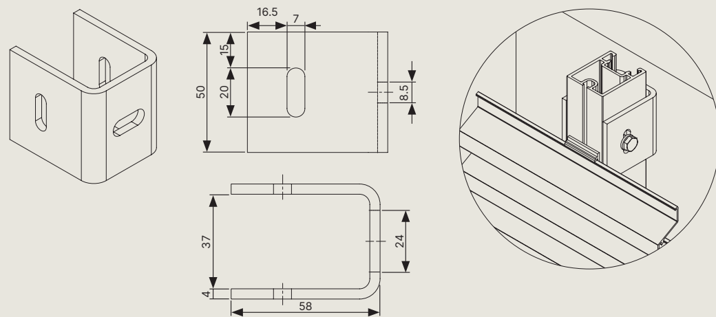
U-bevestigingsbeugel LZ.4210 voor Linius dragers
