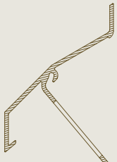
L.050IM1 Lamel met geïntegreerde insectenwering
