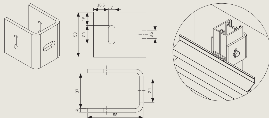
U-bevestigingsbeugel LZ.4210 voor Linius dragers
