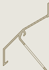
L.050IM1 Lamel met geïntegreerde insectenwering
