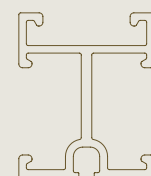
Ref. LD.0440 Voor constructies en zijdelingse bevestiging
