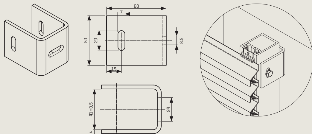
U-bevestigingsbeugel SD.086.11 voor Sunclips dragers
