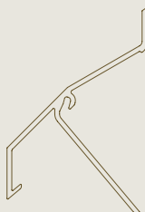
L.050CL Afsluitlamel
