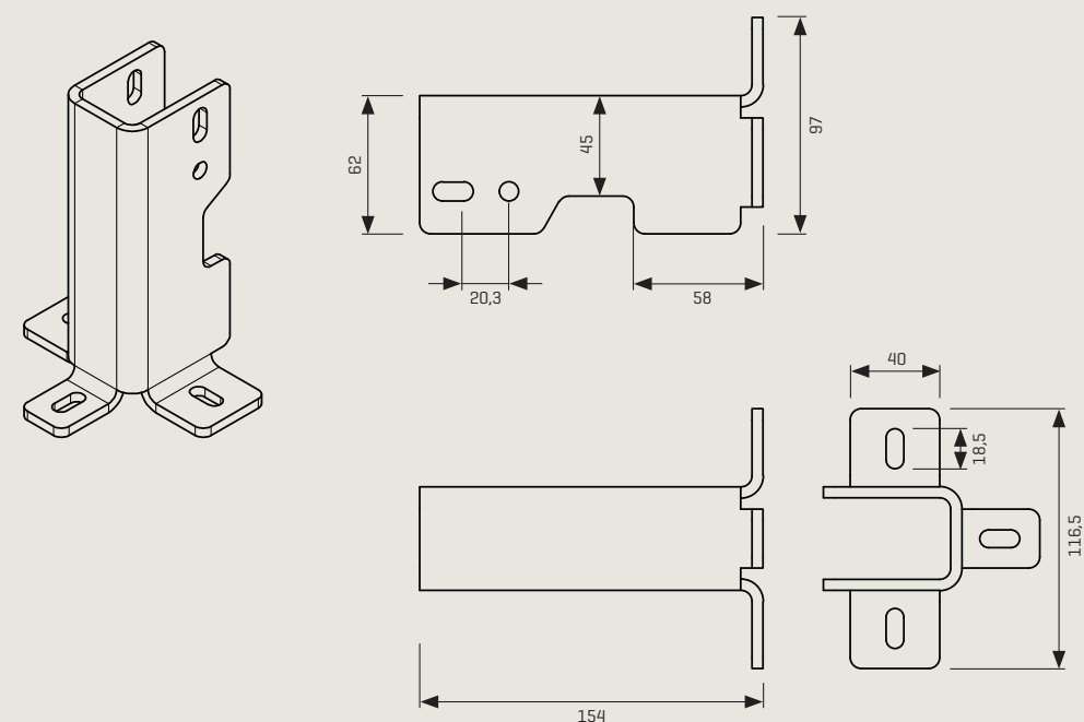
U-bevestigingsbeugel LZ.4215 voor Linius dragers
