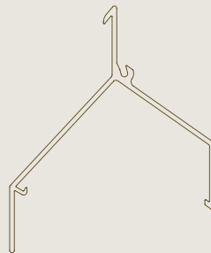
L.066V V-lamel
