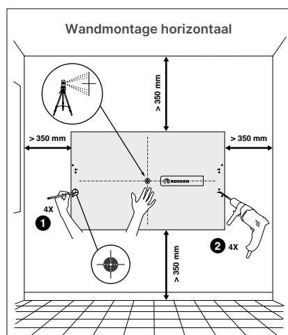
Horizontale wandmontage (met schroeven en pluggen) – gatensjabloon op het boorsjabloon.
