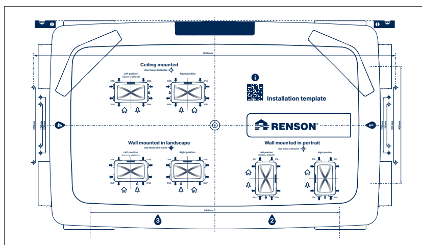
Horizontale wandmontage (met schroeven en pluggen) – gatensjabloon op het boorsjabloon.
