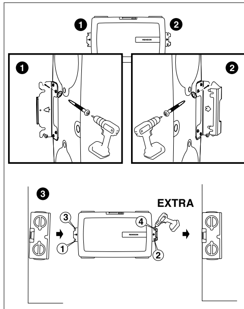
Horizontale wandmontage – Vastgedraaide schroeven.
